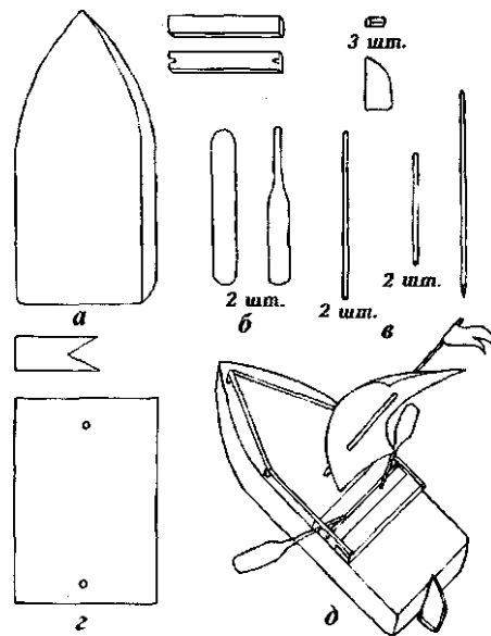
Рис. 135. Човник з вітрилом
