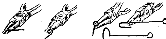
Рис. 83. Згинання дротяної заціпки
