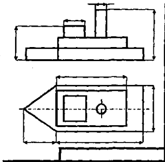
Рис. 17. Креслення моделі кораблика
