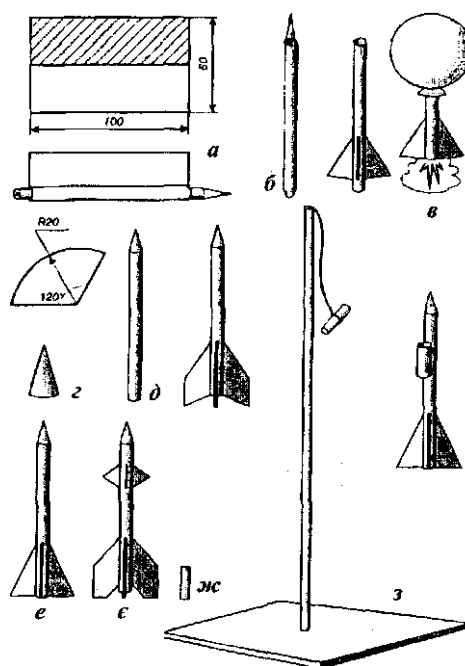
Рис. 132. Моделі ракет
