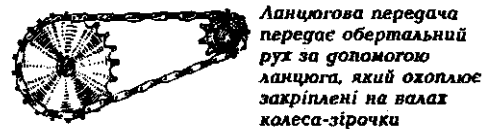
Рис. 116. Ланцюгова передача
