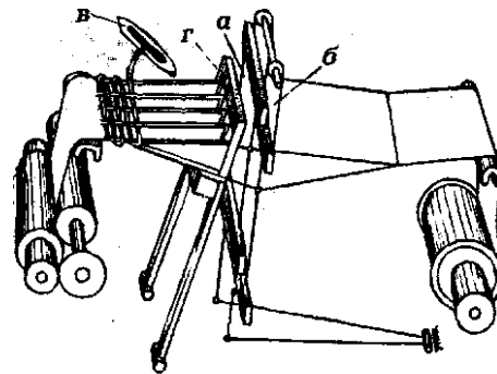
Рис. 55. Схема човникового ткацького верстата
