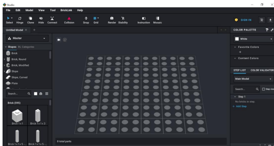
Рис. 2. Інтерфейс Studio 2.0
